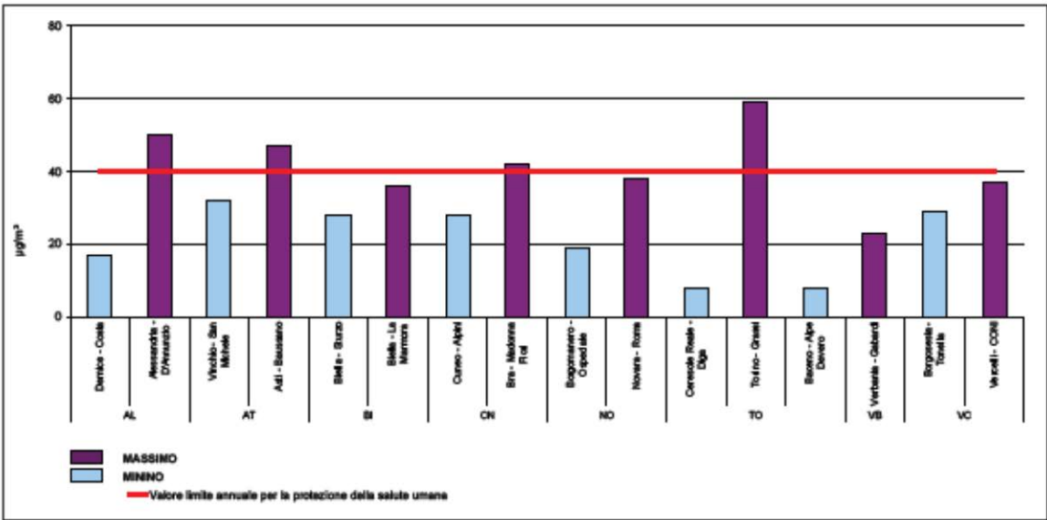
Figura 3.6 - PM 10 , minima e massima media annuale per provincia - anno 2011
