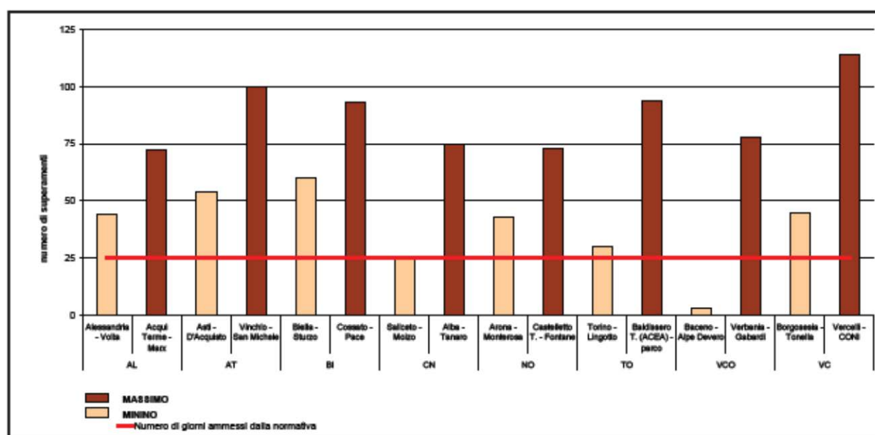
Figura 3.4 - \text{O}_3 , numero minimo e massimo di giorni di superamento del valore obiettivo per la protezione della salute umana per provincia - anno 2011
