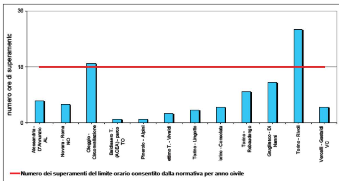
Figura 3.3 - NO 2 , stazioni con almeno un superamento del limite orario di 200 µg/m 3 - anno 2011
